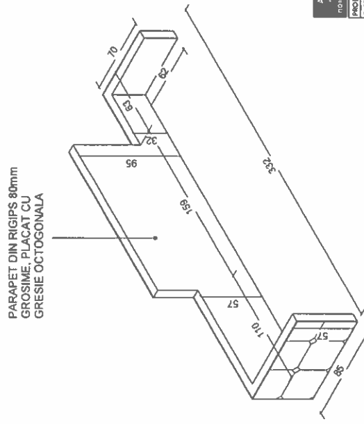
3 axonometrie parapet bar 2
