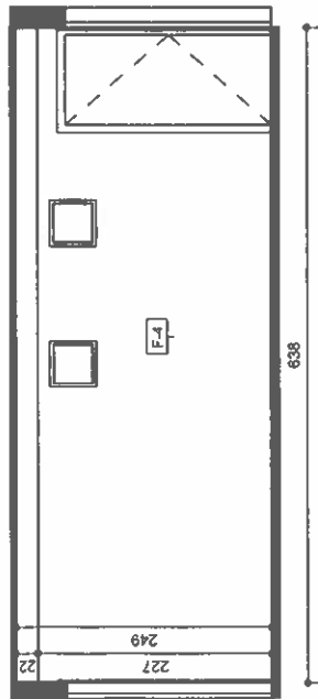
3 Elevatie 2 depozitare/vestiar 1 : 50
