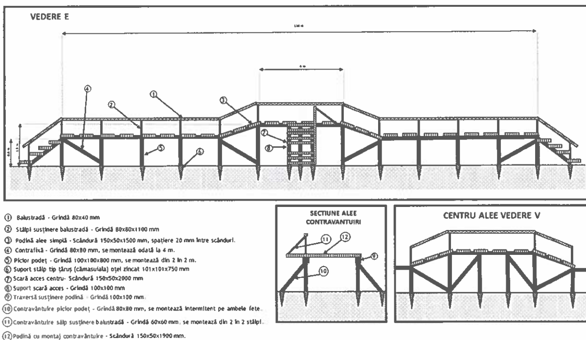
Figura 4.1.: Alee suspendată 1, cu lungimea de 110 m (exemplificare)
