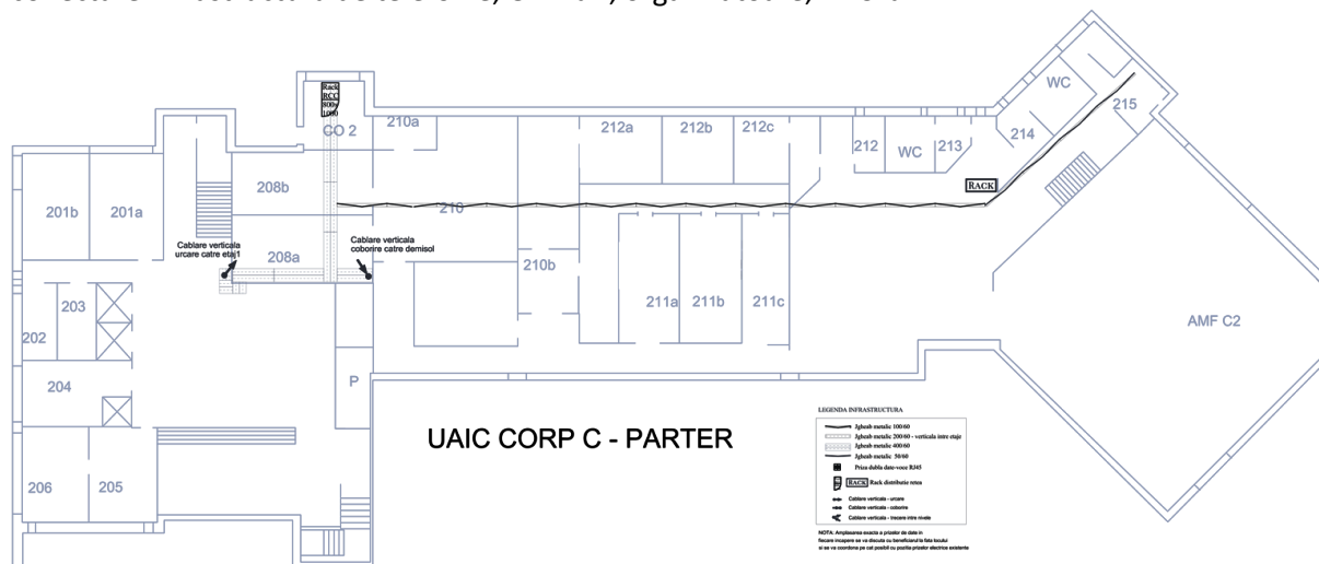
Figura 1. Dispunere rack-uri corp C parter
