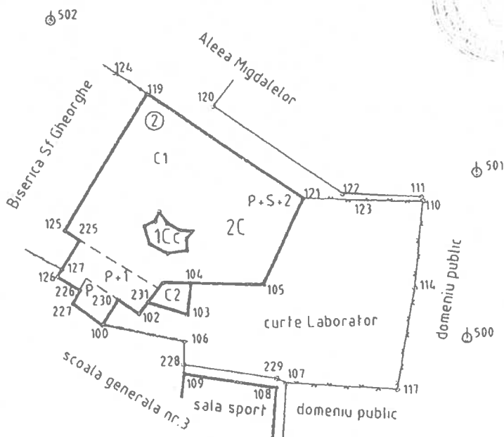
DISTANTE PUNCTE CONTUR IMOBIL
