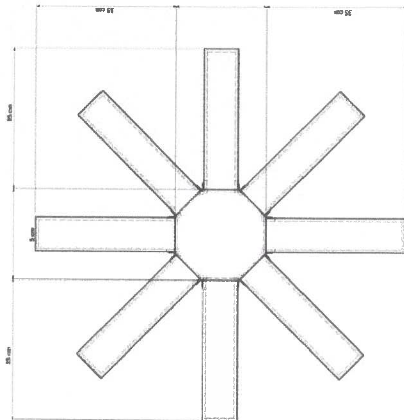
Front view Scale: 1:5
