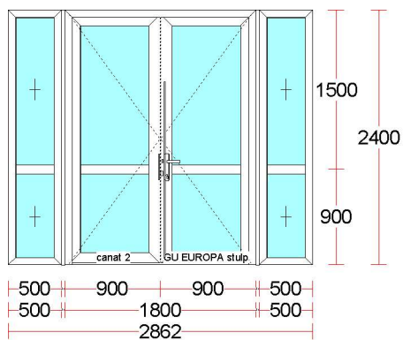
Panou07 - 1 buc.
