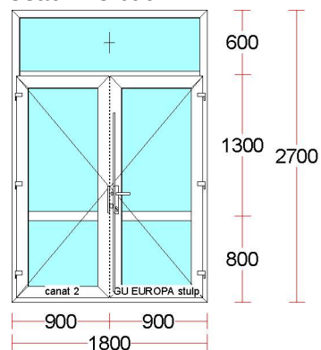
Usa04 - 8 buc.
