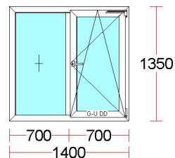
Fereastră02 - 12 buc.
