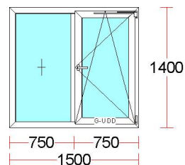
Fereastră06 - 12 buc.
