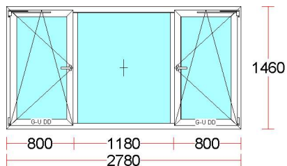
Fereastră01 - 108 buc.
