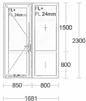
Panou06 - 1 buc.
