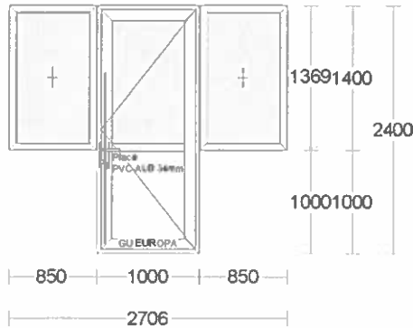
Panou05 - 4 buc.
