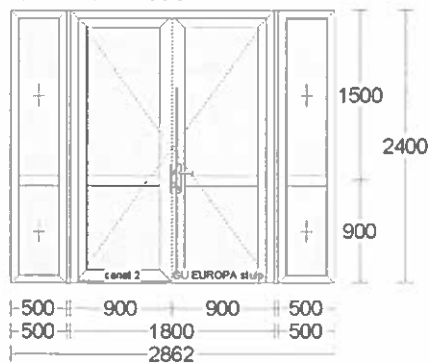
Panou05 - 1 buc.
