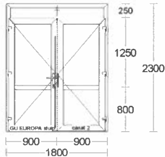
Usa04 - 4 buc.
