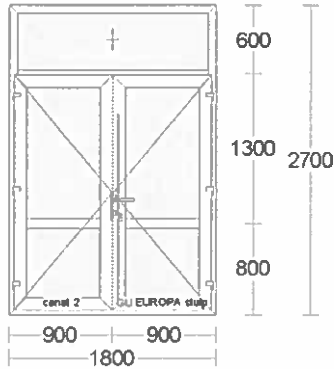
Usa04 - 8 buc.
