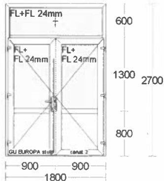
Usa03 - 4 buc.
