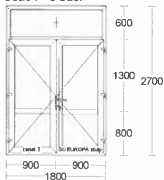
Usa04 - 8 buc.
